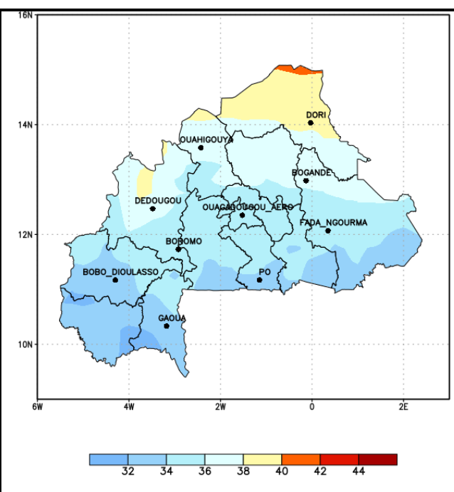
Figure 14 : Températures maximales prévues du 23 au 29 septembre 2023 (Source NOAA GFS)
