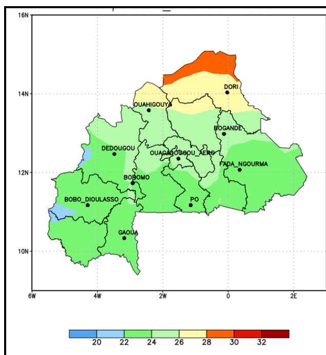
Figure 13 : Températures minimales prévues du 23 au 29 septembre 2023 (Source NOAA GFS)
