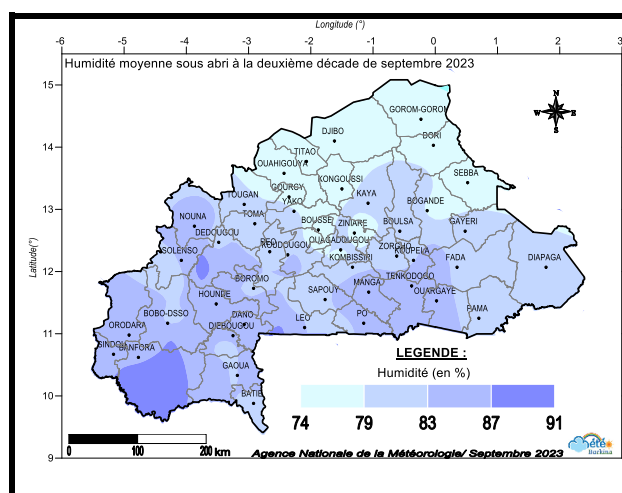
Figure 8 : Evolution de l'humidité relative moyenne à la deuxième décennie de septembre 2023.
