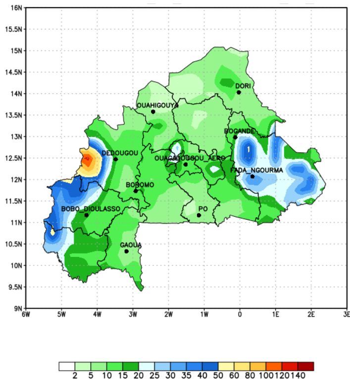
Figure 12 : cumuls pluviométriques prévus du 23 au 29 septembre 2023 (Source NOAA GFS)
