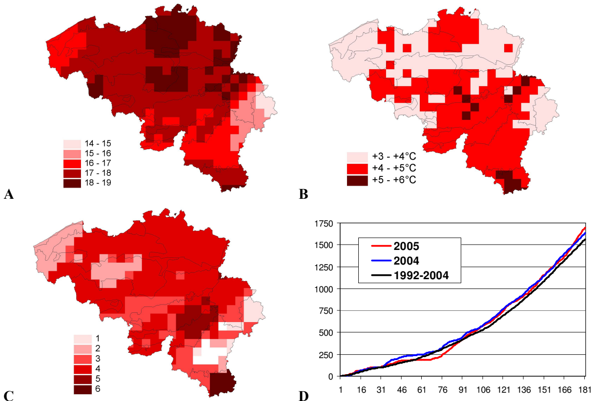
Figure 3 : [A] Température moyenne (°C) mesurée en juin 2005 ; [B] écart de la température (°C) à la moyenne 1992-2004 ; [C] nombre de jours de canicule ( T_{max} > 30^{\circ}\text{C} ) observés en juin 2005 ; [D] évolution de la somme des températures positives de janvier à juin 2005 en Hesbaye par rapport à 2004 et à la moyenne 1992-2004.
