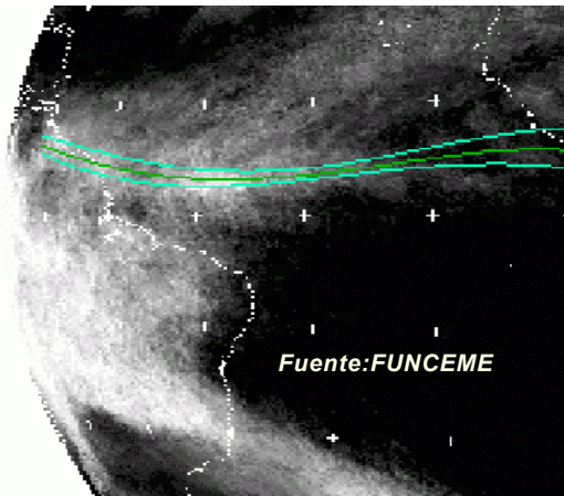
Figura 6. Posición promedio de la ZCIT en el Atlántico tropical para la última semana de diciembre del 2003
