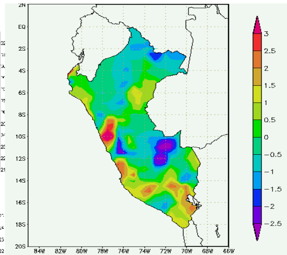
Mapa 1. Anomalías de la Temperatura Máxima (°C) Diciembre 2003
