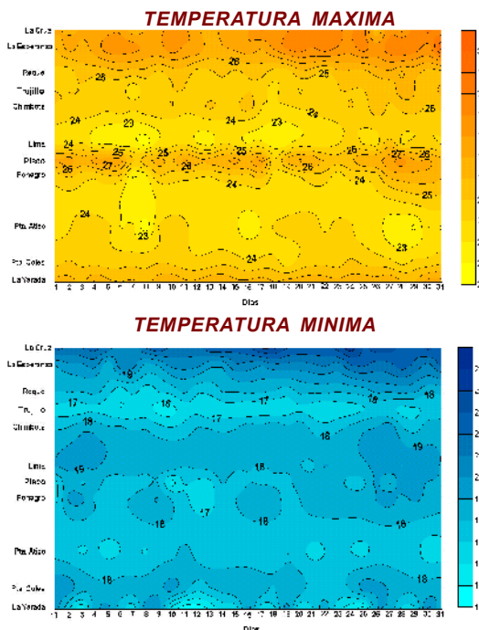
Figura 13. Temperaturas extremas del aire en estaciones costeras (°C)
