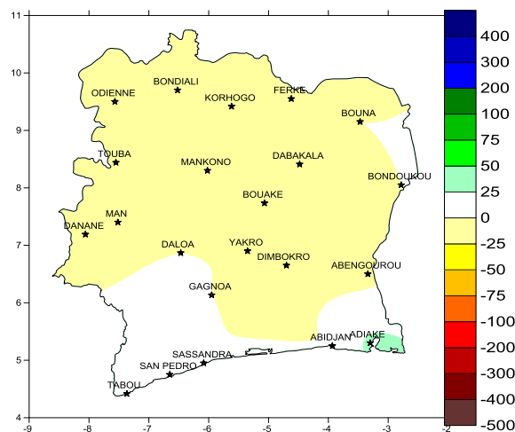
Fig2 : Ecarts entre la pluviométrie (mm) du 1 au 10 janvier 2017 et du 1 au 10 Janvier 2016
