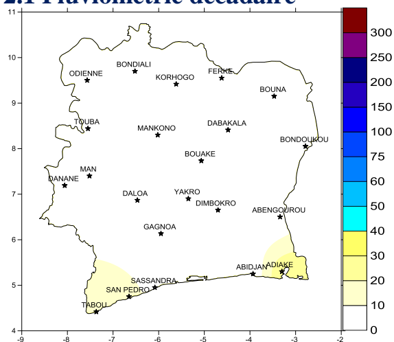
Fig1 : Pluviométrie totale (mm) du 1 au 10 janvier 2017
