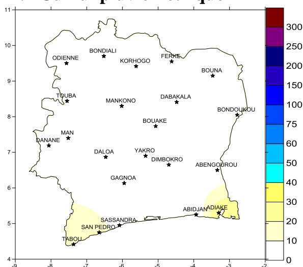
Fig 3 : Cumul pluviométrique (mm) du 1 au 10 Janvier 2017
