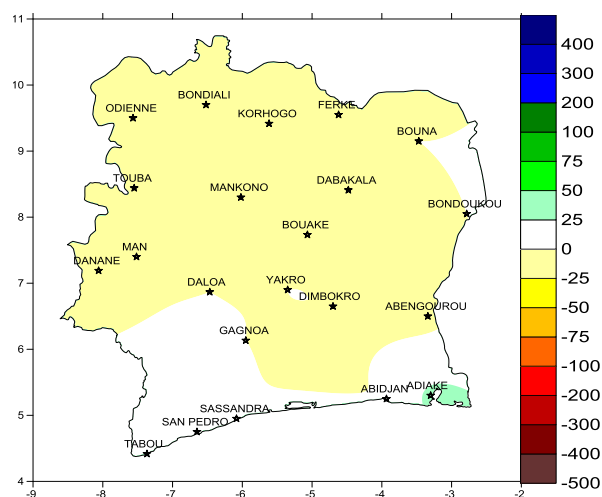
Fig 4 : Ecart entre Cumuls pluviométriques du 1 au 10 Janvier 2017 et du 1 au 10 Janvier 2016
