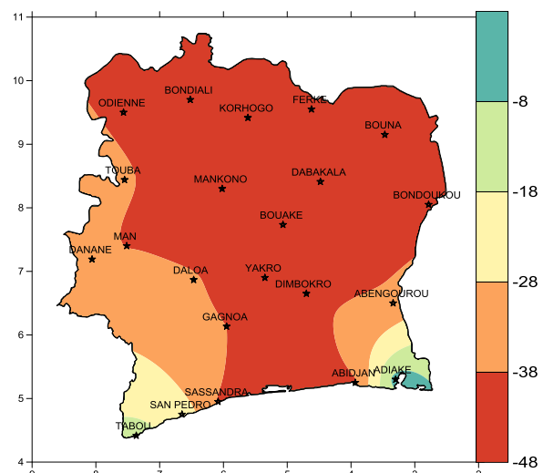
Fig 9 : Bilan hydrique climatique (mm) du 1 au 10 Janvier 2017
