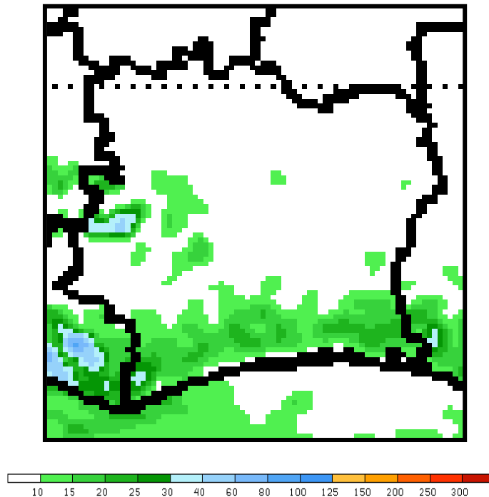
Figure 10 : prévision de la pluviométrie du 17 au 24 Janvier 2017 (source : NOAA, climat Prédiction Center)
