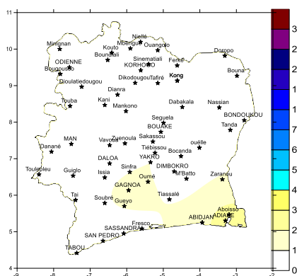
Fig1 : Pluviométrie décadaire (mm) du 21 au 31 Déc. 2020
