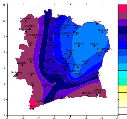
Fig. 3 : Cumul pluviométrique (mm) du 1 Janvier au 31 Déc. 2020
