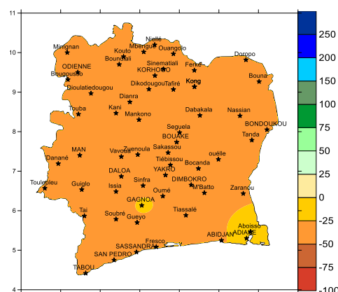
Fig. 9: Bilan hydrique climatique (mm) du 21 au 31 Déc. 2020
