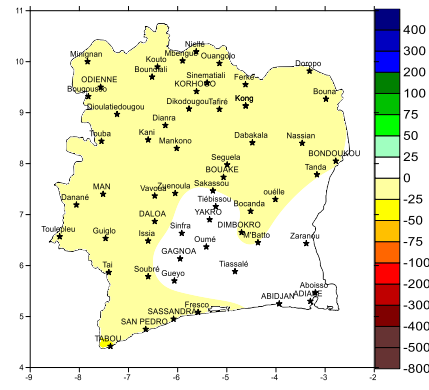
Fig2 : Ecart entre la pluviométrie (mm) du 21 au 31 Déc. 2020 et du 21 au 31 Déc. de la normale (1981-2010)
