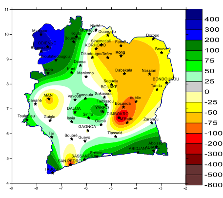
Fig. 4 : Ecart entre Cumuls pluviométriques du 1 Janvier au 31 Déc. 2020 et du 1 Janvier au 31 Déc. de la normale (1981-2010)
