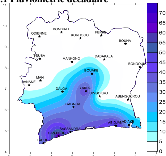
Fig1 : Pluviométrie totale (mm) du 01 au 10 Décembre 2016
