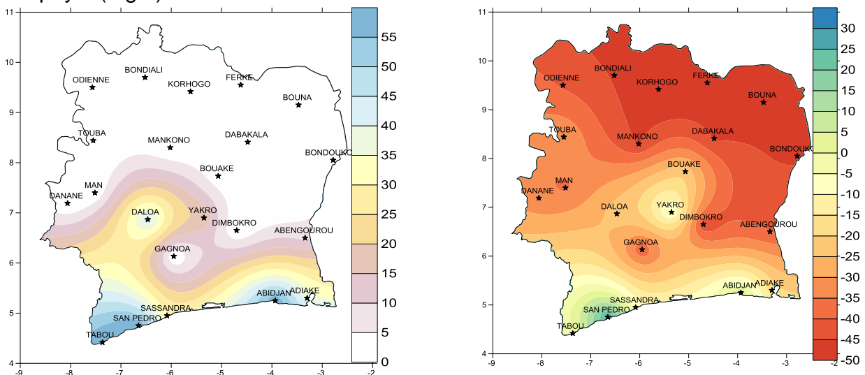
Fig. 9 : Bilan hydrique climatique (mm) du 01 au 10 Décembre 2016
