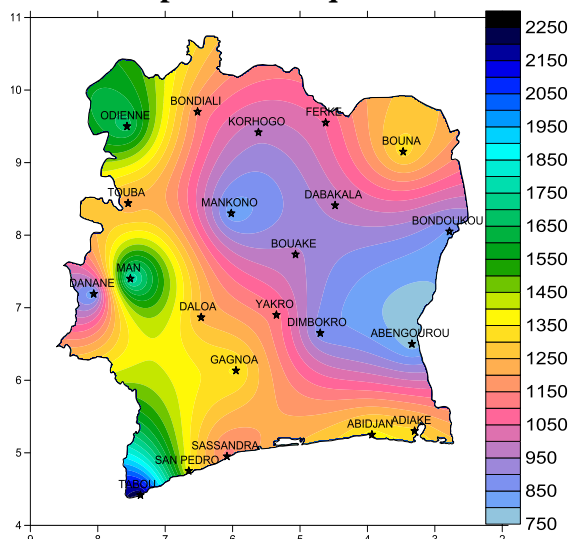
Fig 3 : Cumul pluviométrique (mm) du 1 janvier au 10 Décembre 2016
