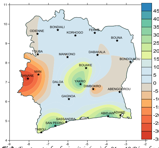
Fig2 : Ecart entre la pluviométrie (mm) du 01 au 10 Décembre 2016 et du 01 au 10 Décembre 2015
