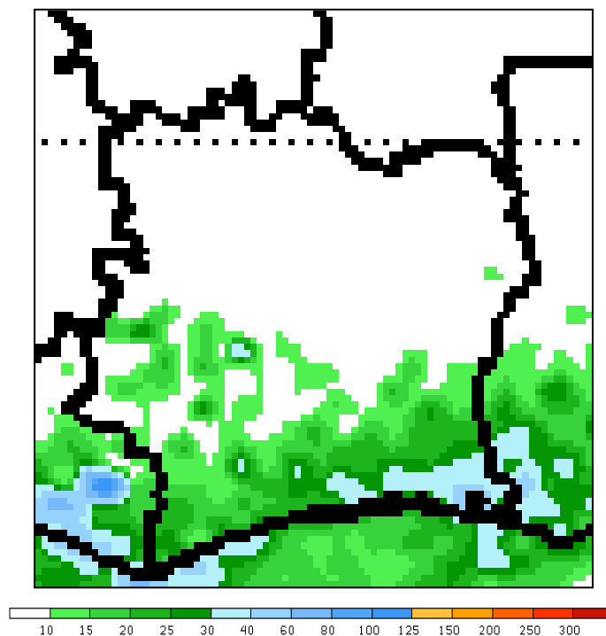
Figure 10 : prévision de la pluviométrie du 15 au 22 Décembre 2016 (source : NOAA, climate Prédiction Center)
