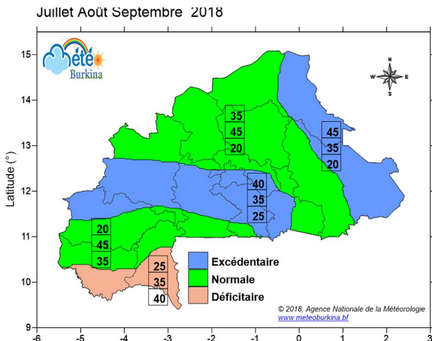
Figure 17 : Prévion saisonnière du cumul pluviométrique JAS 2018
