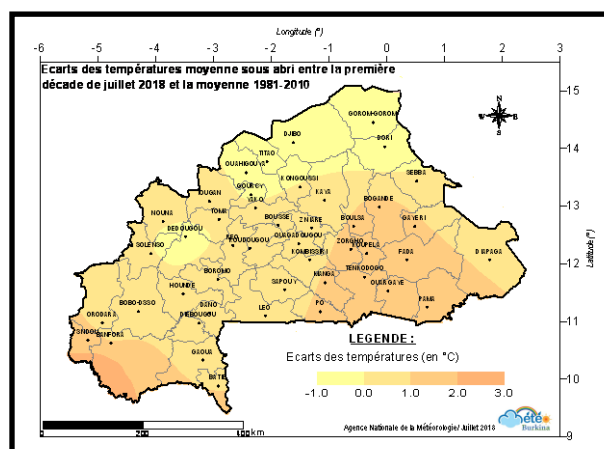
Figure 7 : Ecart des températures moyennes de la première décade de juillet 2018 et la moyenne (1981-2010).
