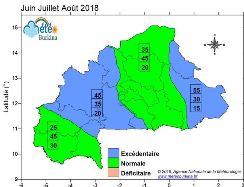
Figure 16 : Prévision saisonnière du cumul pluviométrique JJA 2018
