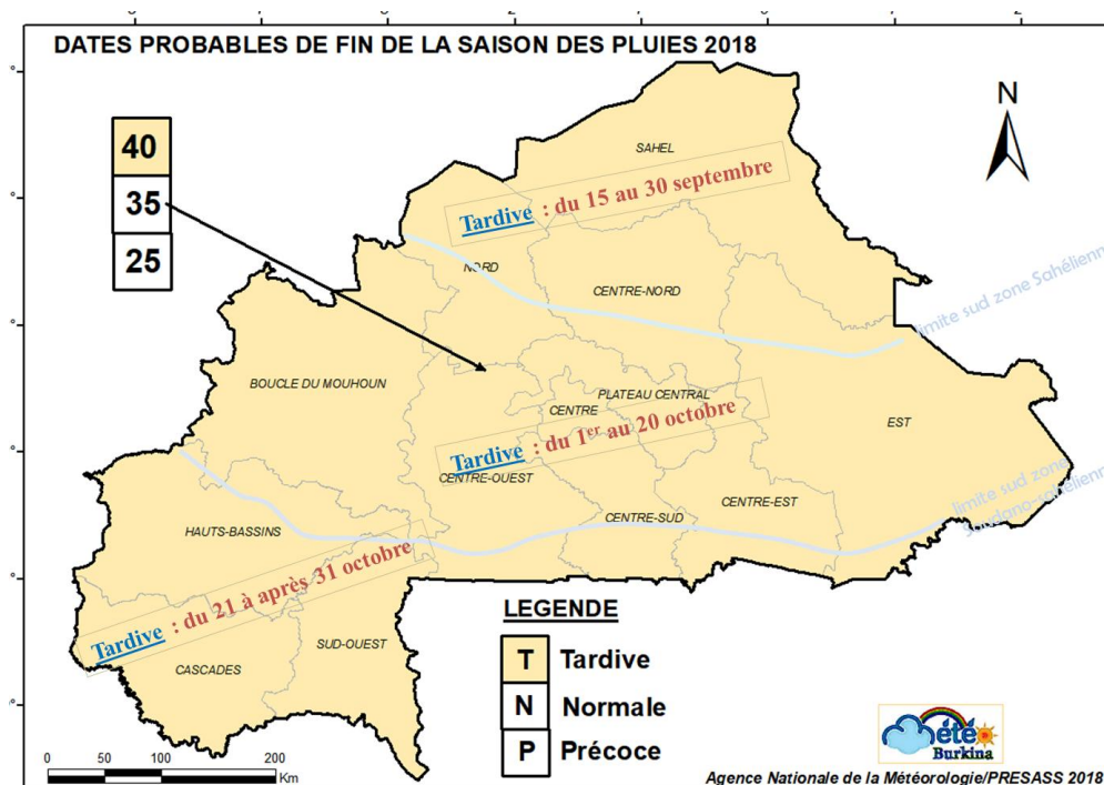
Figure 19 : Tendances probables des dates de fin de la saison des pluies 2018
