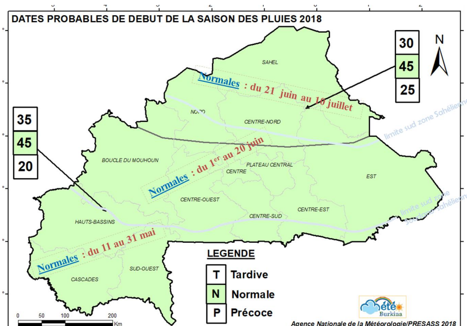
Figure 18: Tendances probables des dates de début de la saison des pluies 2018
