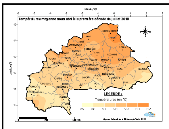
Figure 6 : Températures moyennes sous abri à la première décade de juillet 2018.
