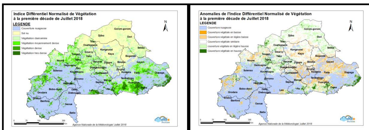
Figure 12a : Indice Différentiel Normalisé de Végétation à la première décennie de juillet 2018.
