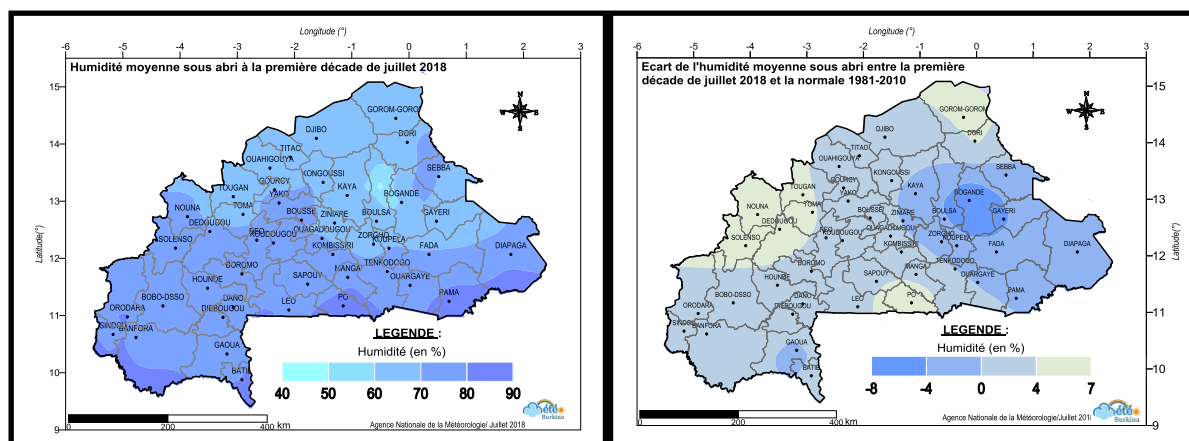
Figure 8 : Evolution de l'humidité relative moyenne à la première décennie de juillet 2018.
