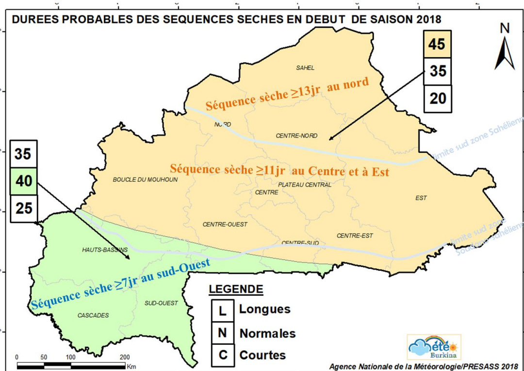
Figure 20 : Durées probables des séquences sèches en début de saison des pluies 2018
