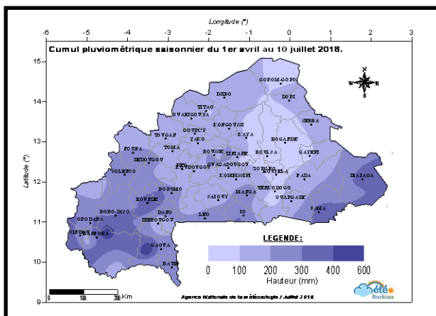
Figure 3 : Cumul pluviométrique saisonnier du 01 avril au 10 juillet 2018.
