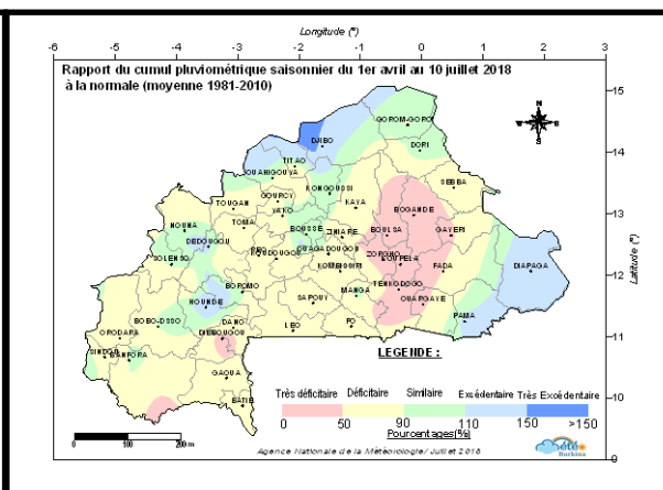
Figure 4 : Rapport du cumul pluviométrique du 1 er avril au 10 juillet 2018 à la normale 1981-2010.
