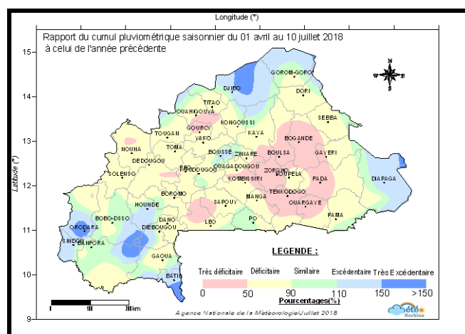
Figure 5 : Rapport du cumul pluviométrique du 1 er avril au 10 juillet 2018 à celui de l'année précédente.
