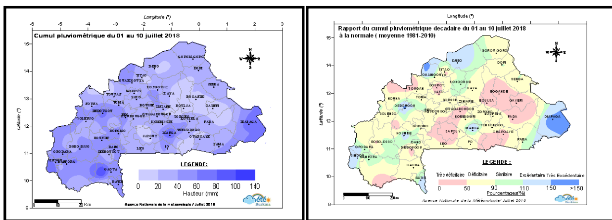
Figure 1 : Cumuls pluviométriques à la première décade de juillet 2018.
