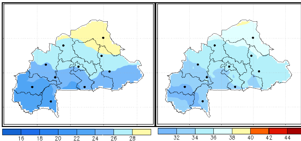
Figure 14 : NOAA GFS : Températures minimales prévues du 12 au 18 juillet 2018
