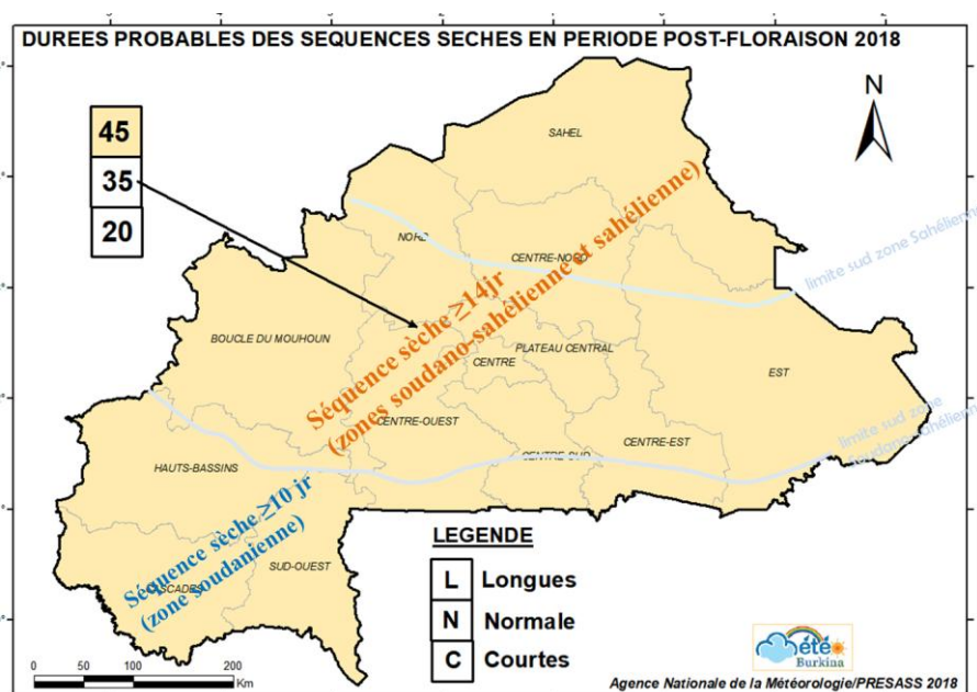
Figure 21 : Durées probables des séquences sèches en fin de saison des pluies 2018
