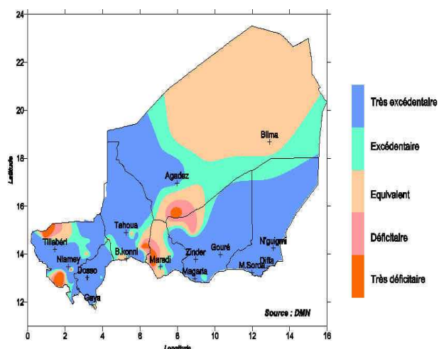
Fig 2 : cumul pluviométrique au 30 septembre ecart par rapport à 2011
