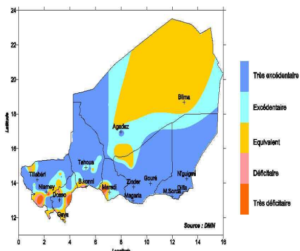
Figure 4 : cumul pluviométrique au 30 septembre ecart par rapport à la Moyenne 1981_2010
