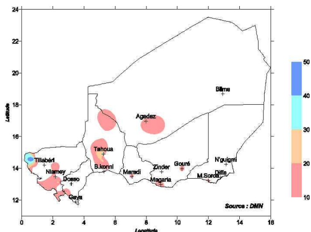
Fig 1 : pluviométrique 3 Emme décade septembre 2012
