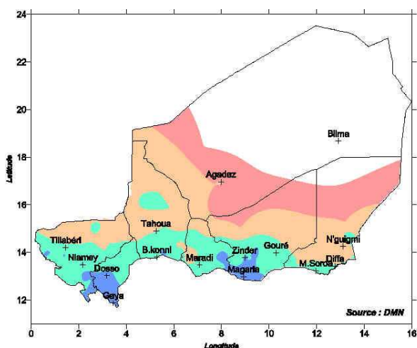
Figure 3 : cumul pluviométrique au 30 septembre 2012
