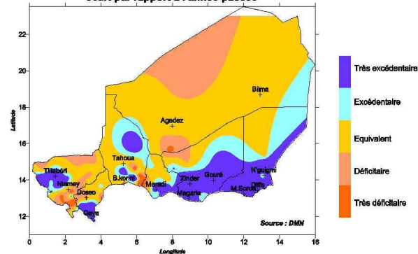
Fig.4: Pluviométrie cumulée au 20 Juillet 2012 écart par rapport à la moyenne 1981_2010
