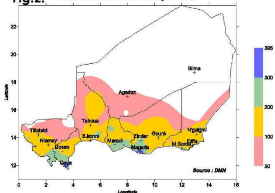
Fig.2: Pluviométrie cumulée au 20 Juillet 2012
