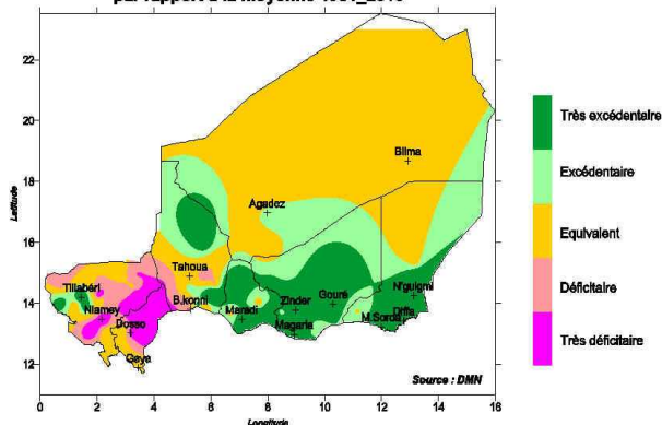
Fig.4: Pluviométrie cumulée au 20 Juillet 2012 écart par rapport à la moyenne 1981_2010
