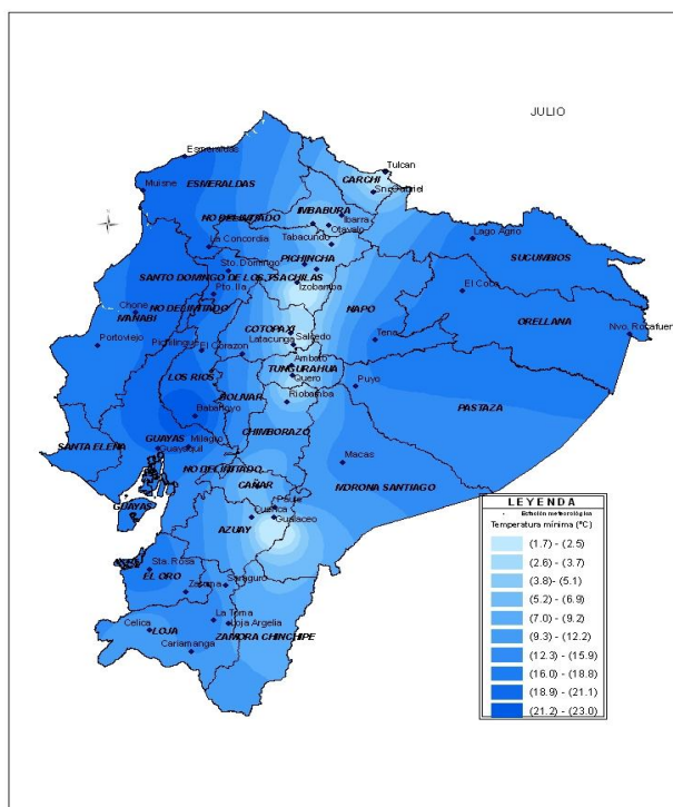
Gráfico 2. Distribución de la temperatura mínima en el mes de julio
