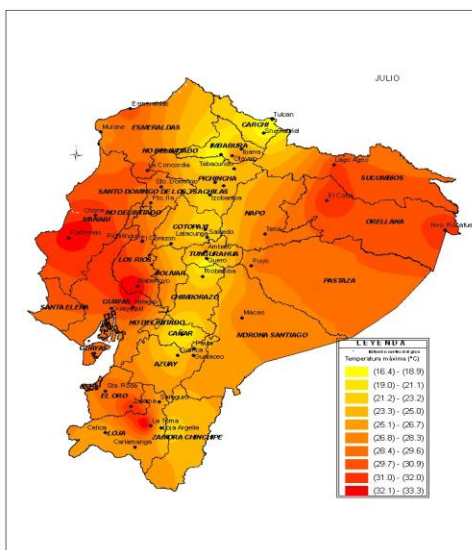
Gráfico 3. Distribución de la temperatura máxima en el mes de julio
