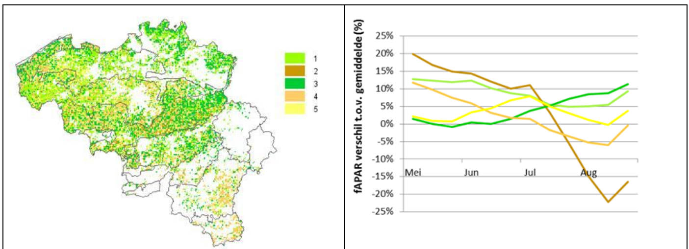
Figure 2: Classification des zones cultivées (5 classes) établie à partir de l'évolution de la différence de fAPAR au cours de 3 derniers mois avec les valeurs normales sur cette même période.
